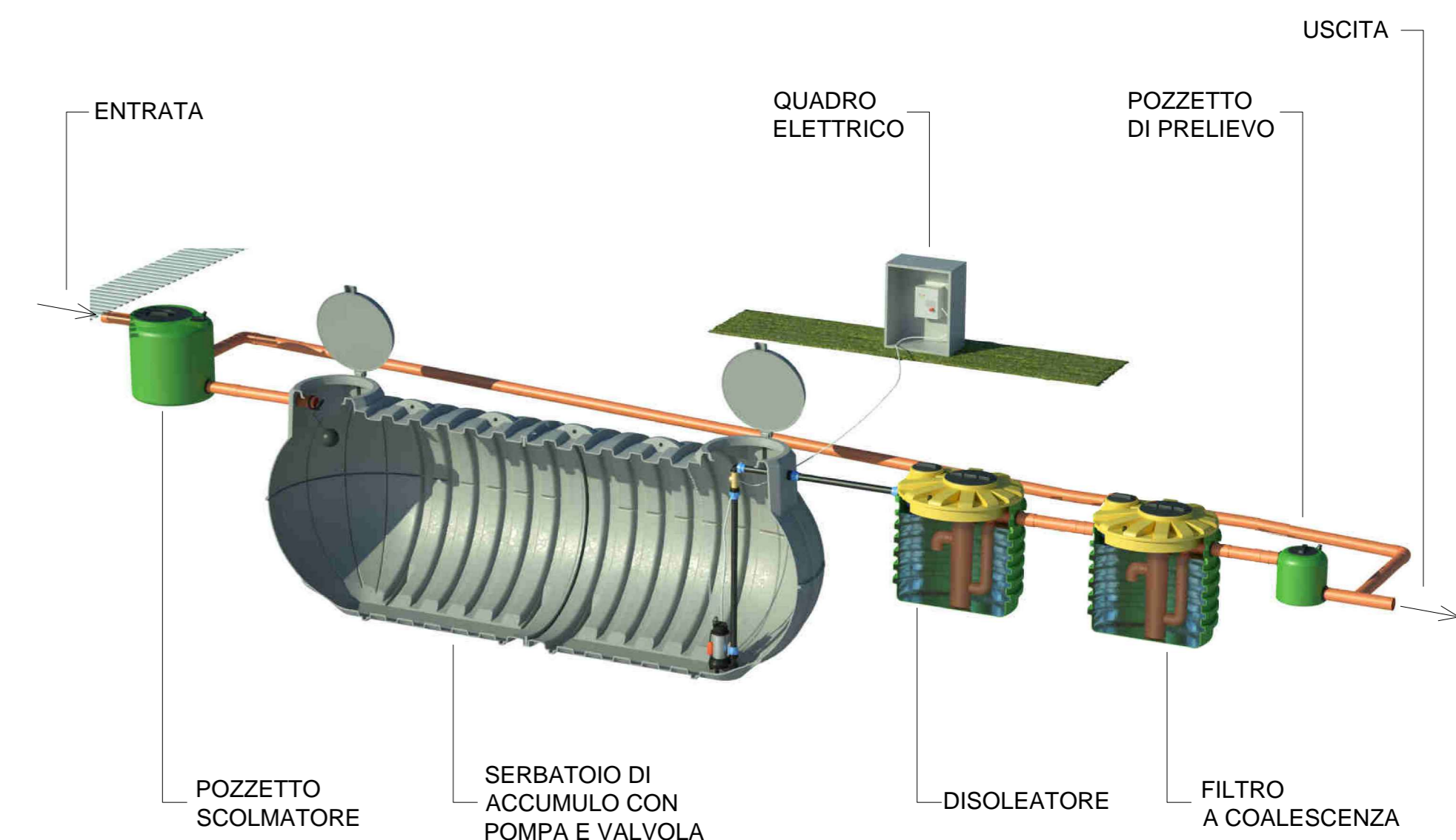
Impianto di stoccaggio prima e seconda pioggia interrato, e pozzetto di prelievo campioni
